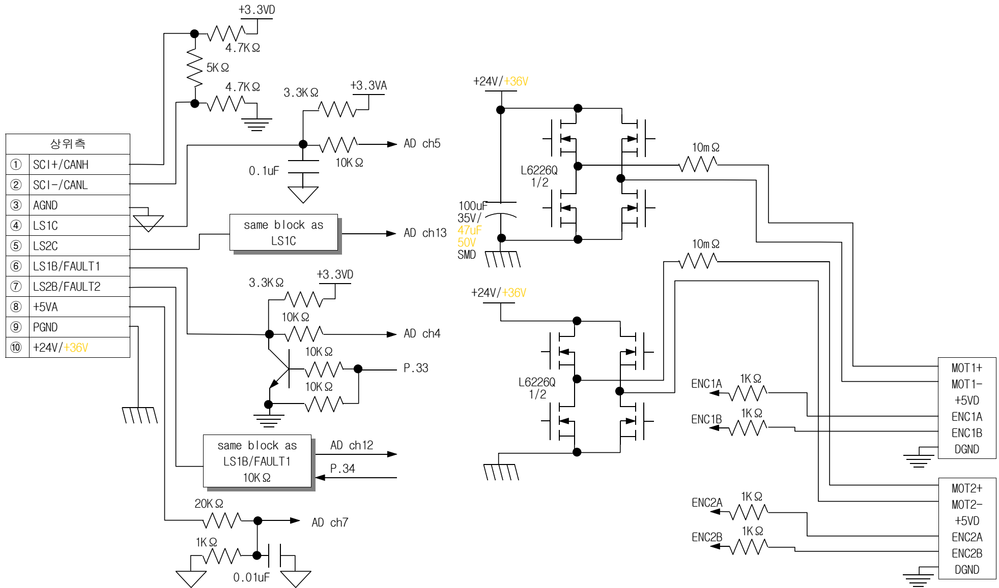
CUBE-DC2401-DIQ의 입출력 내부회로
