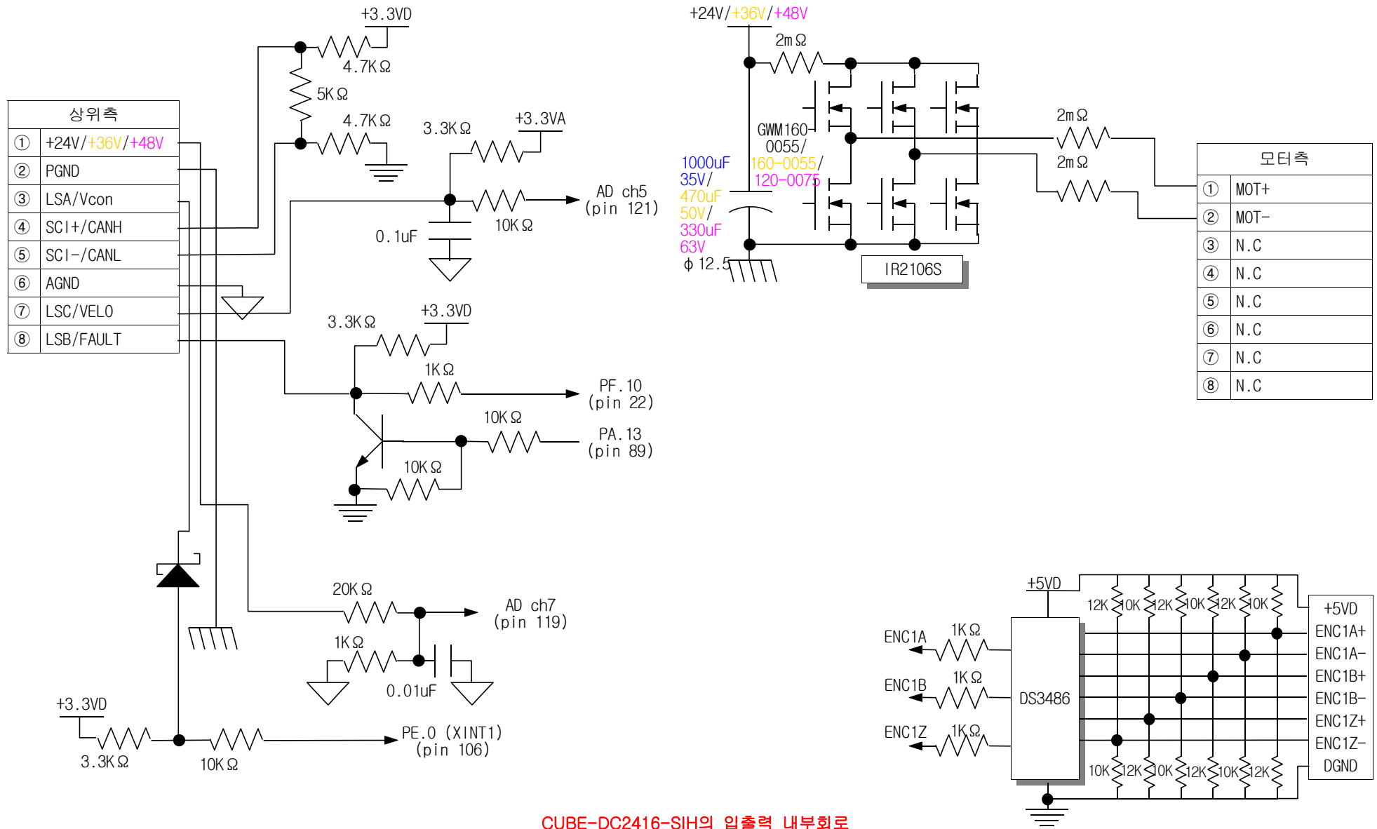
CUBE-DC2416-SIH의 입출력 내부회로
