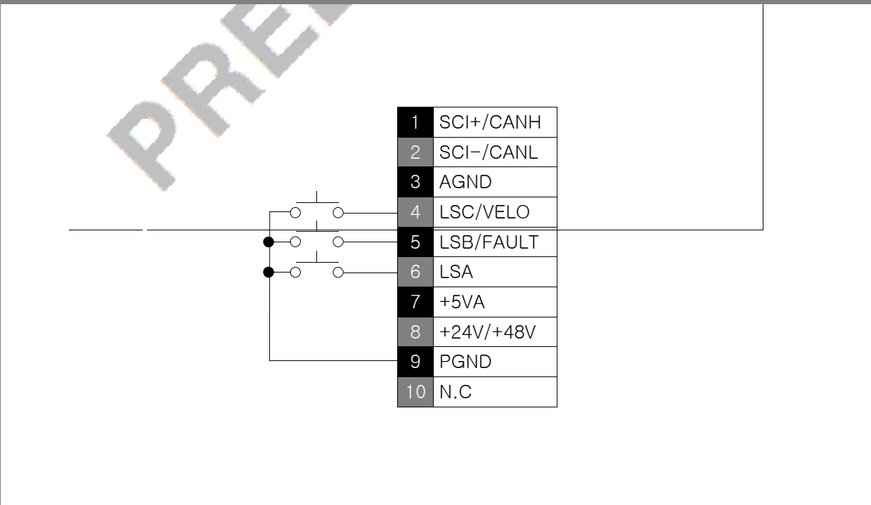
CUBE-DC24xx-Sxx SERIES (모든 포트를 디지털 입력으로 사용할 때)
